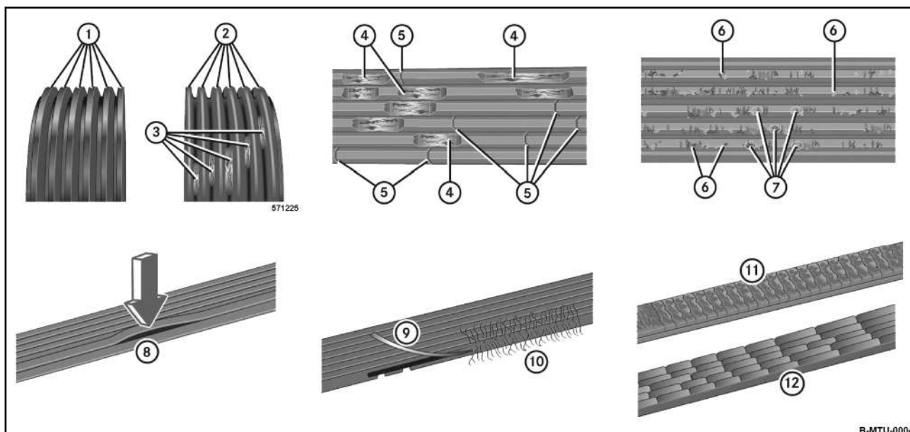
Fig. 210: Imágenes de daño correa trapezoidal con dentado interior.
