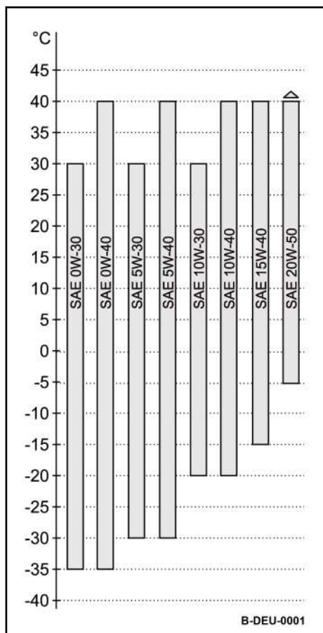
Fig. 168: Diagrama de viscosidad de aceites
